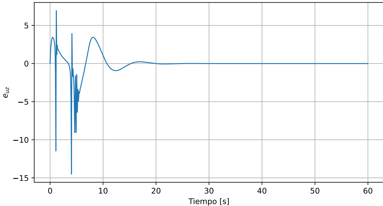
Error de seguimiento con paso: uz
